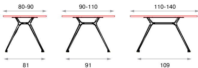
Размеры столешниц и опор
