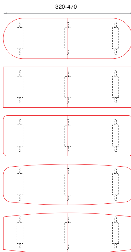
Столы составные линейные
