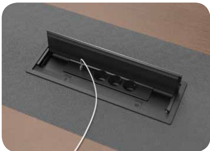
Лючок для вывода проводов с двусторонним открыванием в комплекте с розеточным блоком: 3 силовые розетки + USB (A+C) + Cat6 + HDMI, кабель питания 1,8 м
